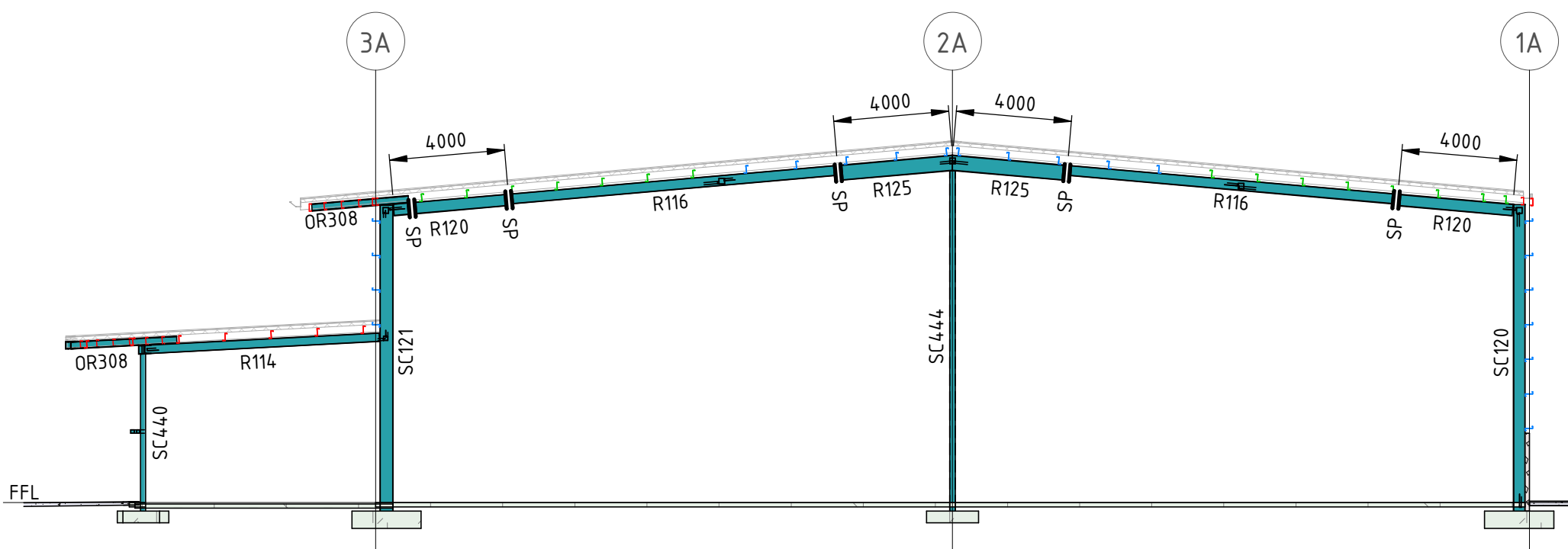
SECTION A7 SCALE 1 : 200
