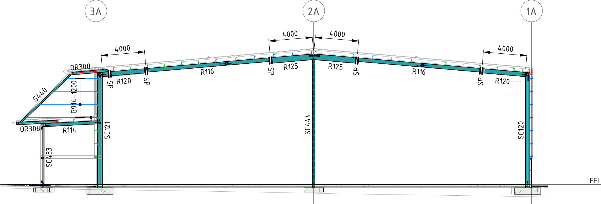
SECTION A6 SCALE 1 : 200
